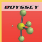
VSEPR Theory
